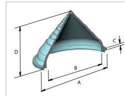
GROMMET
